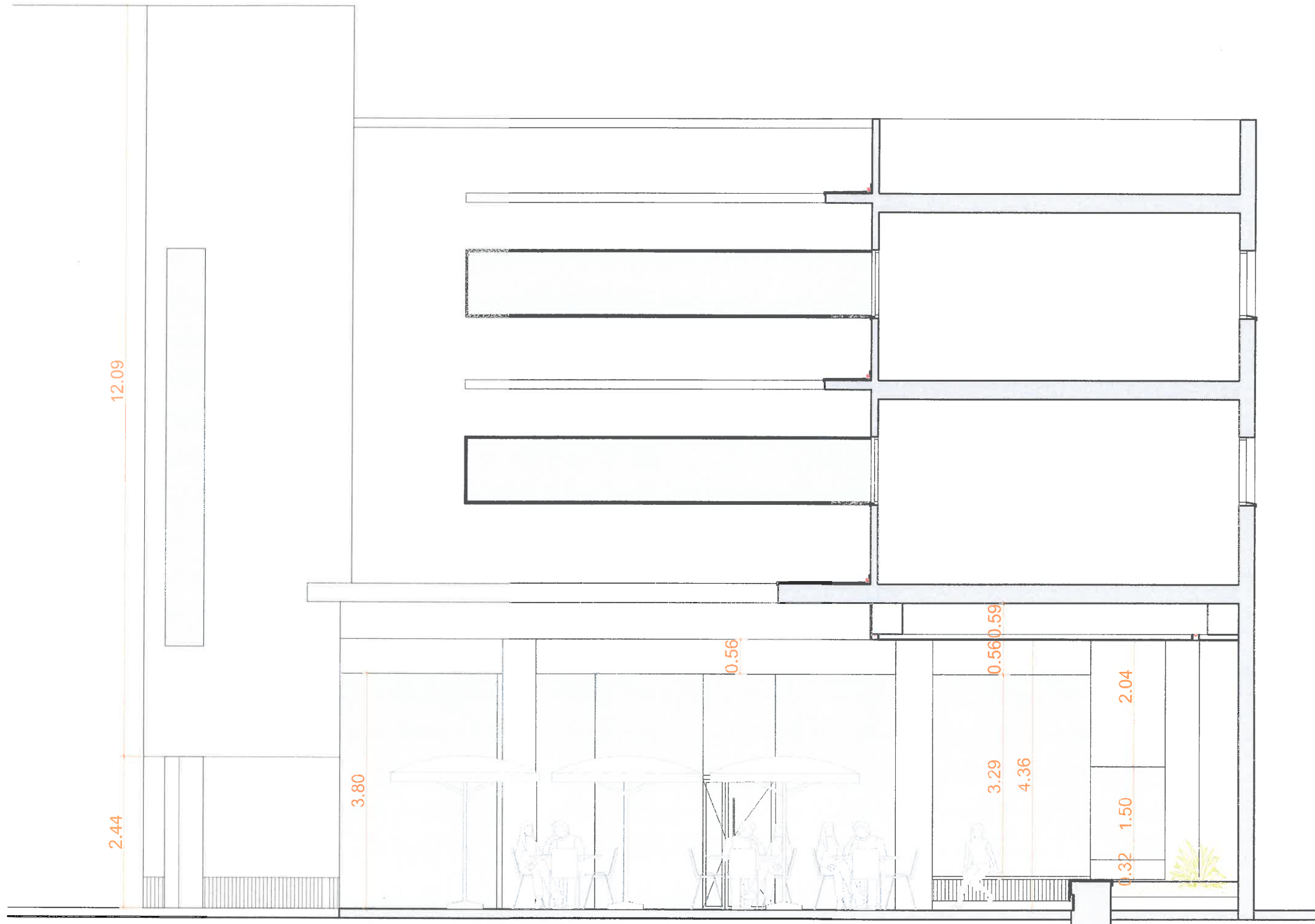
SECCIÓN TRANSVERSAL
