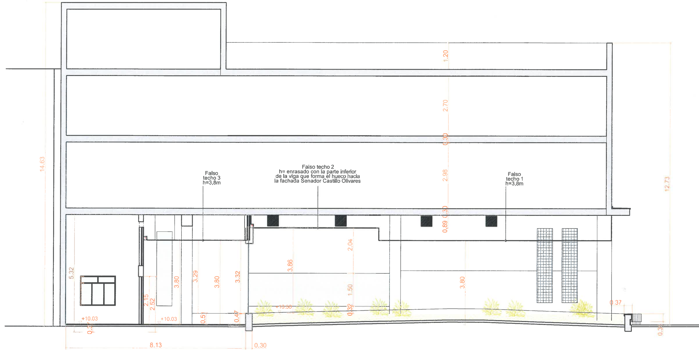
SECCIÓN LONGITUDINAL
